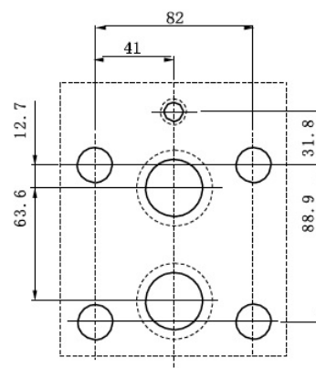
МКПВ-32
