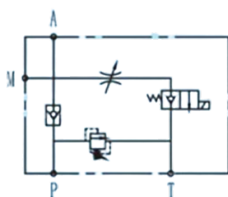
EV...NC
