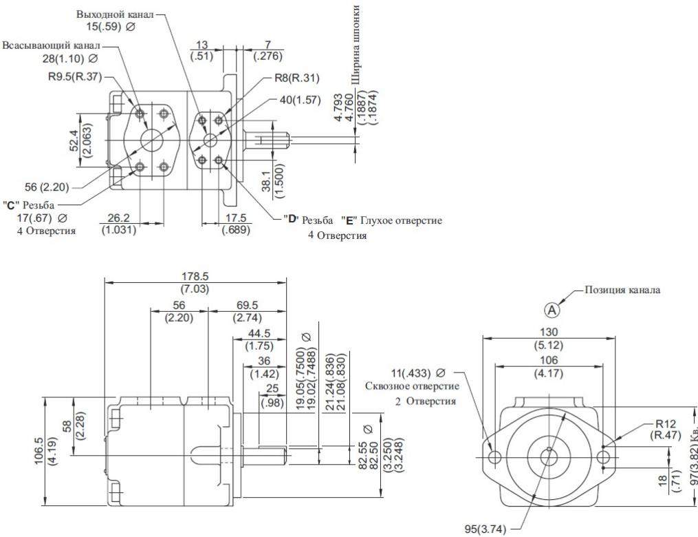
Чертеж насоса PV2R1-19
