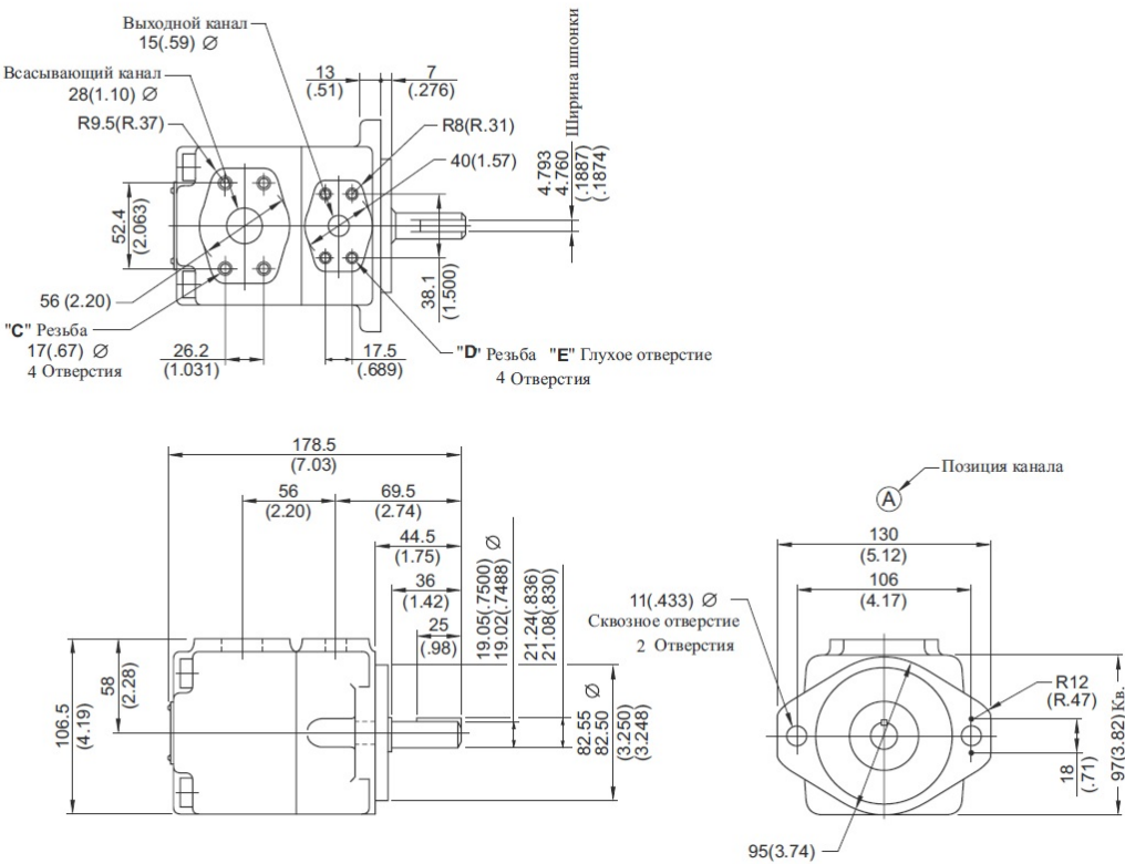
Чертеж насоса PV2R1-8
